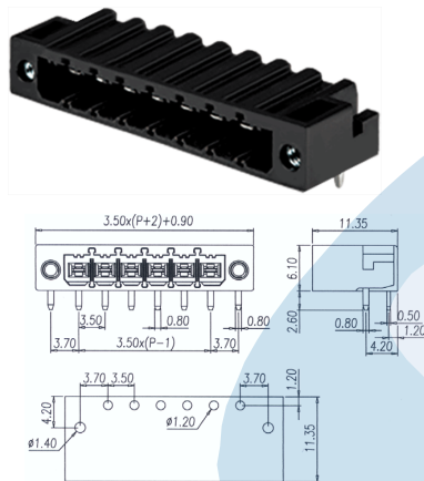
P/N: BC022516-XX-TH
