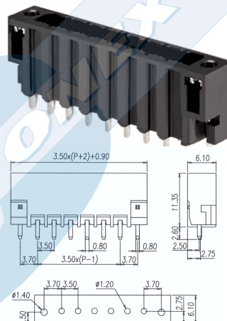
P/N: BC022517-XX-TH
