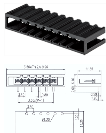
P/N: BC022526-XX-TH
