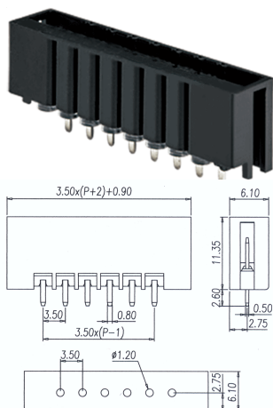
P/N: BC022527-XX-TH
