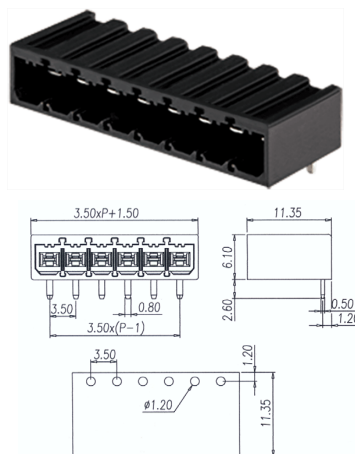
P/N: BC022536-XX-TH
