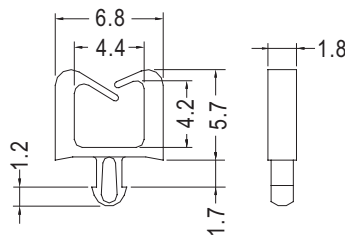
P.C.B Ø1.75 THICKNESS 1.6
