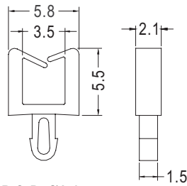
P.C.B Ø2.0 THICKNESS 1.6~1.8
