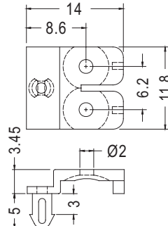
P.C.B Ø3.0
