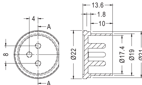
剖面圖 A-A
