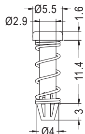
P.C.B Ø3.0
