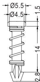
P.C.B Ø3.0
