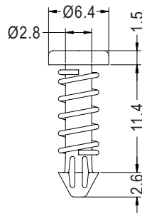
P.C.B Ø3.0
