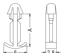
P.C.B Ø3.0
