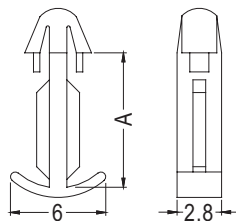
P.C.B Ø3.0
